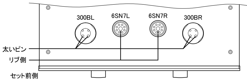
真空管部を上から見た図
