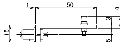
主要寸法図
